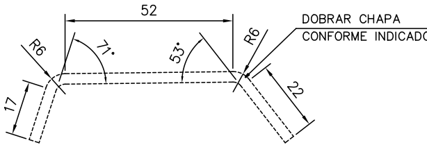
DETALHE SUPORTE DE APOIO(03)
