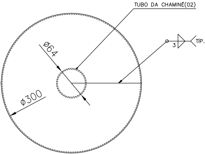
SUPERIOR
