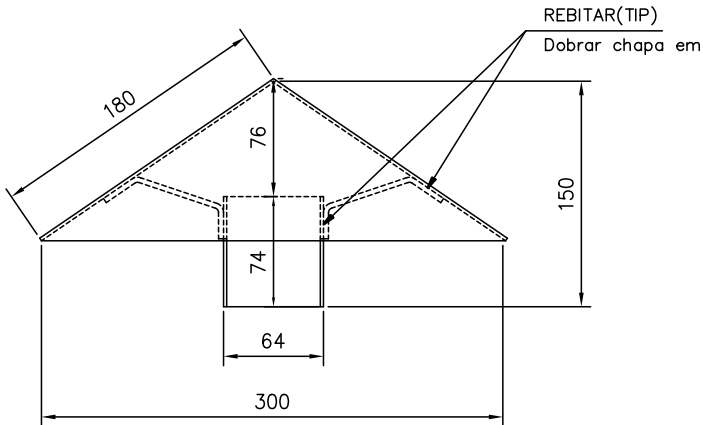
FRONTAL
